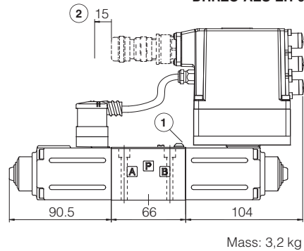
DHRZO-AES-EH-012
