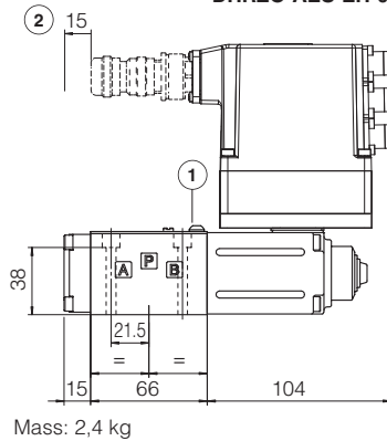
DHRZO-AES-EH-010
